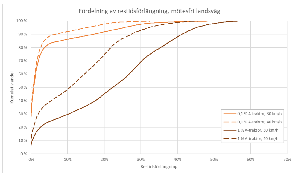
Figur 18: Fördelning av restidsförlängning för övrig trafik på mötesfri landsväg med en hastighetsgräns på 100 km/tim.
