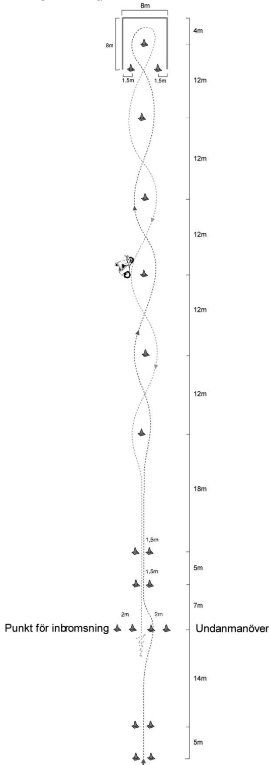
Figur 2. Manöverprovets högfartsdel
