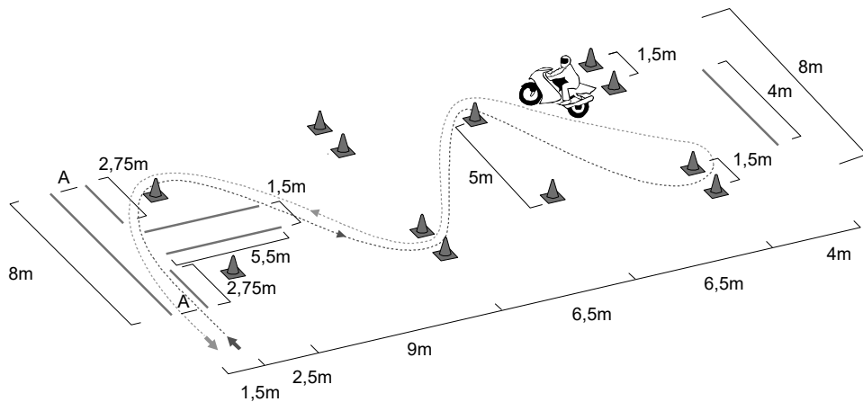
Figur 1. Manöverprovets lågfartsdel
